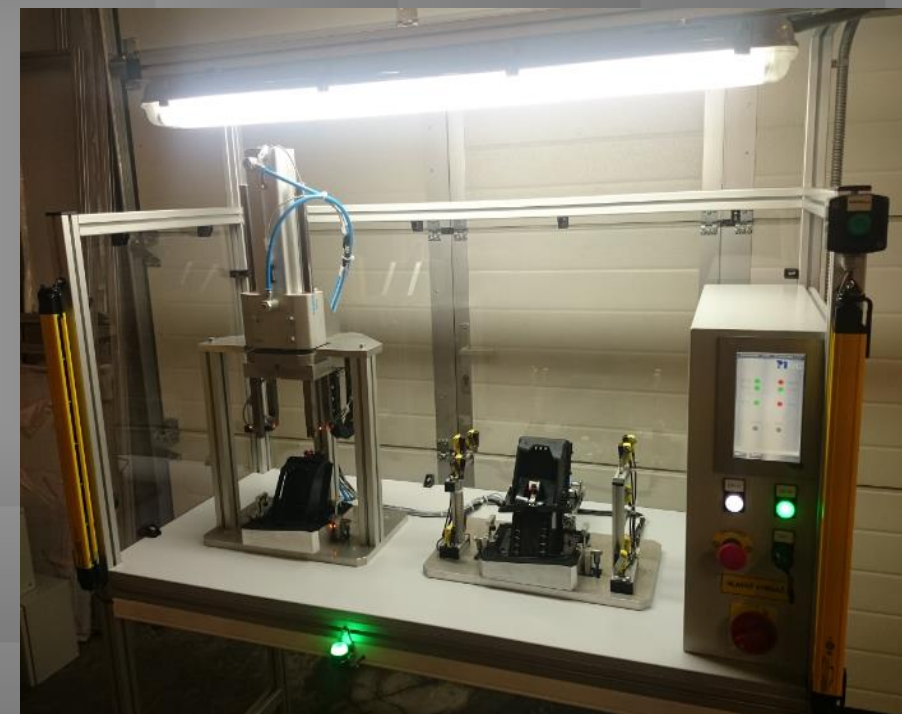
Lisovacie/kontrolné pracovisko
